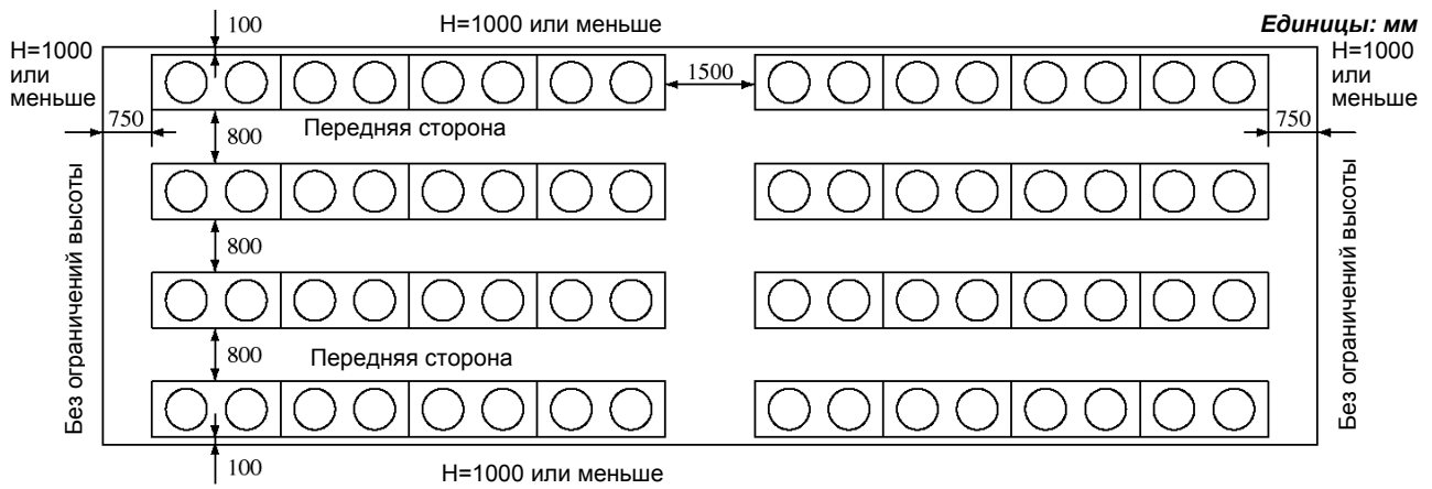
③ [Пример 1] Множество блоков установлено вертикальными и горизонтальными рядами
