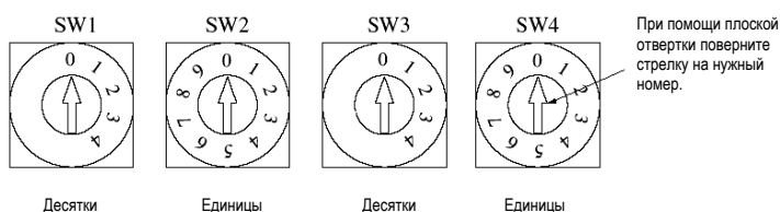
Поворотные переключатели внутреннего блока (SW)
