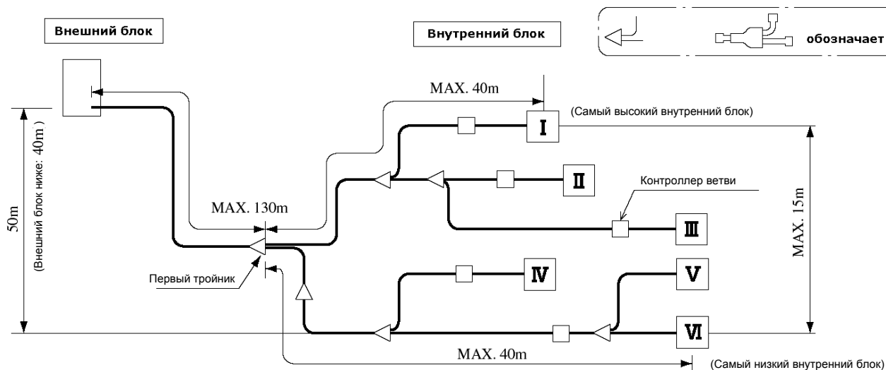
Допустимая длина трубопровода, перепад высот между внутренним и внешним блоками
