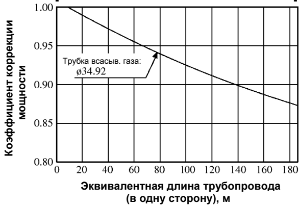
Модель FDCA850HKXRE4 [FDCA400HKXRE4 + FDCA450HKXRE4]
